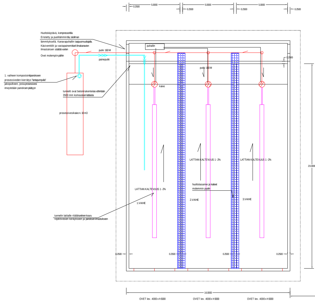
KOMPOSTOINTIRAKENNUS, TOIMINTAKAAVIO, PERIAATEPIIRROS JA PÄÄMITAT
